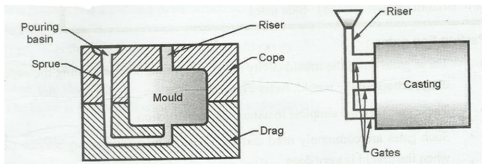
Fig. 1.36 Bottom gate
