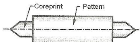
Fig. 1.30 : Core print
