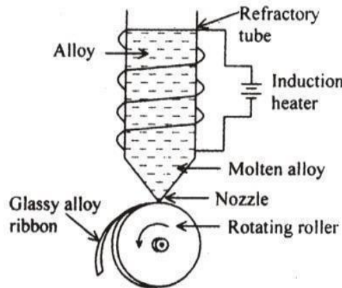
Fig:4.1.1- Melt spinning technique
