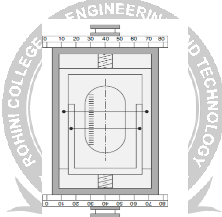
Subtense diaphragm
