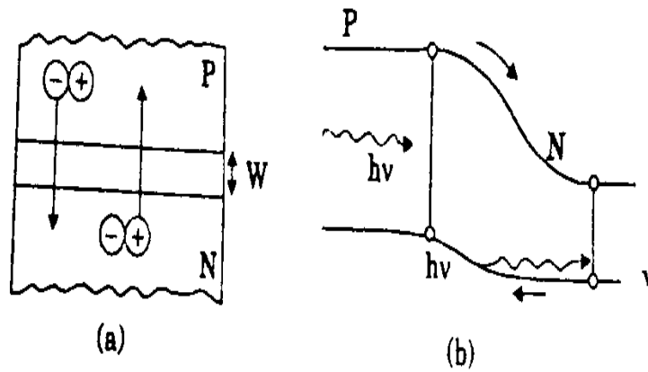
Fig 4.4.2. Energy band
