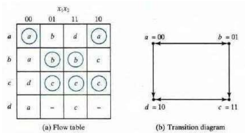
Fig 4.5.9 – a).Flow Table, b).Transition diagram
