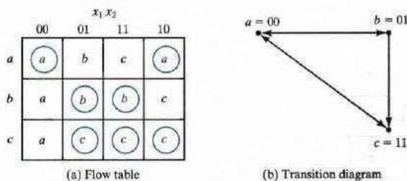
Fig 4.5.8 – a).Flow Table, b).Transition diagram
